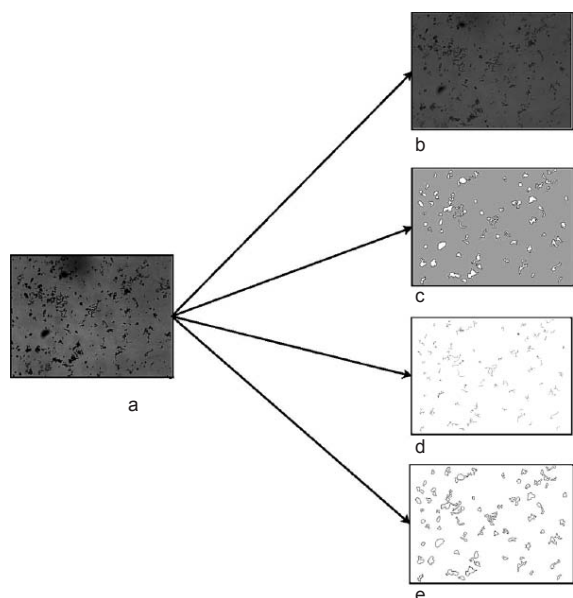
Figura 3. (0) Desenfoque gaussiano (1) conversión a Escala de gris. Procesamiento de imagen: (a) imagen original formato RGB – Input del software , las imágenes de salida del software son (b) imagen en escala de gris (c) imagen trinarizada (d) imagen de esqueletos de los objetos (e) imagen de bordes
